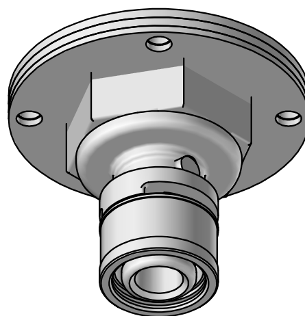
参考斜視図
